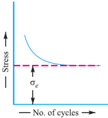
Fig. 4 Endurance/fatigue limit
